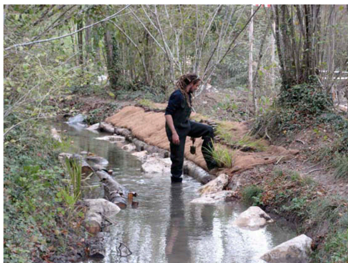
Plantations de végétation aquatique par l'entreprise Sitel sur le tronçon des Eaux-Froides réaménagé. La section du ruisseau a été réduite, notamment à l'aide de blocs qui offrent des abris pour les poissons - novembre 2006.
