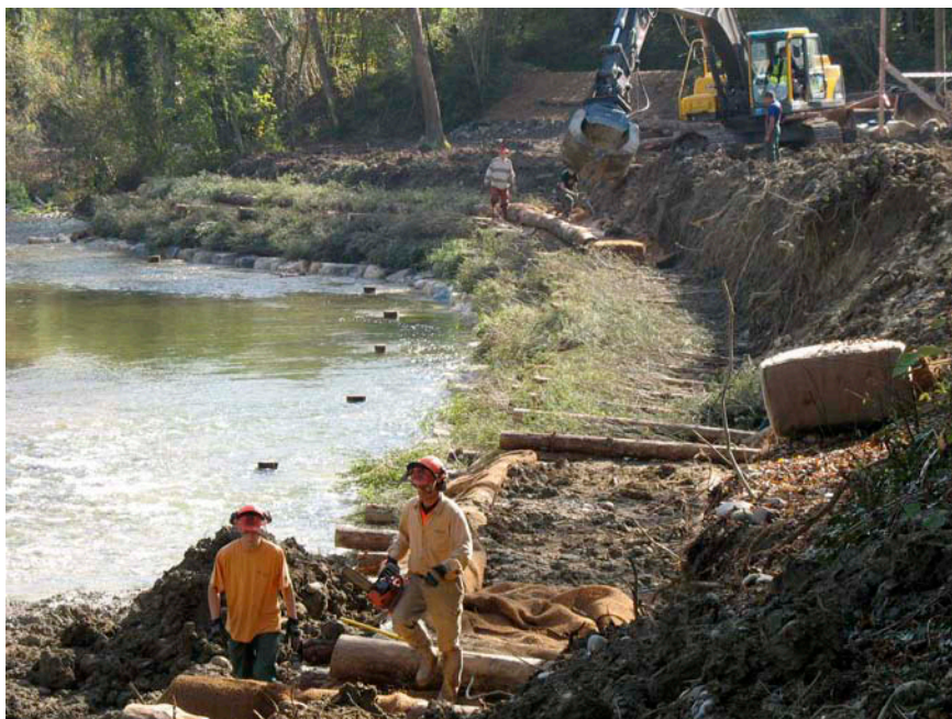
Construction du caisson végétalisé par les apprentis forestiers-bûcherons du DT et par l'entreprise Rampini - octobre 2006.
